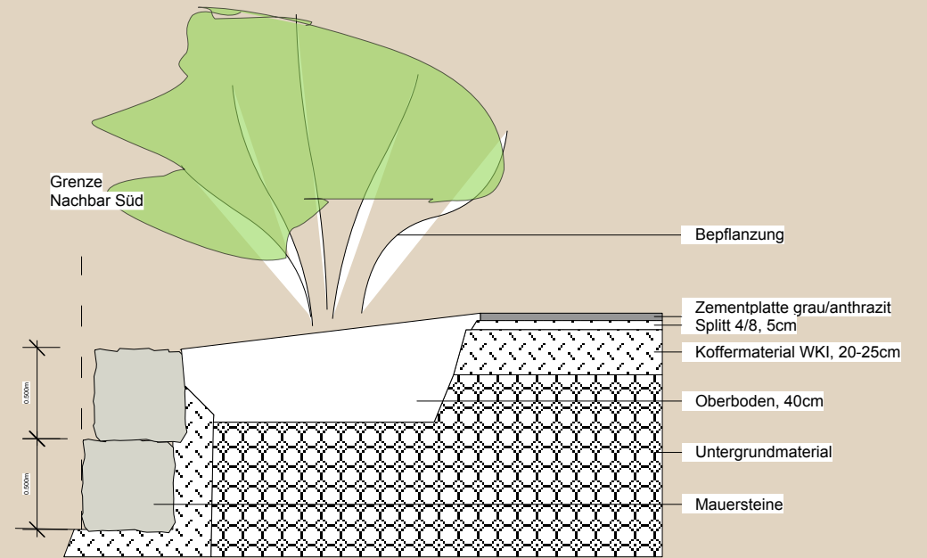
Schnitt A:A'
